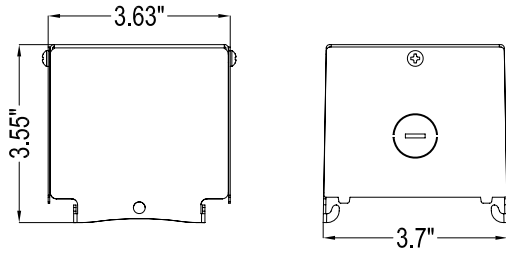
Pendant Mount
